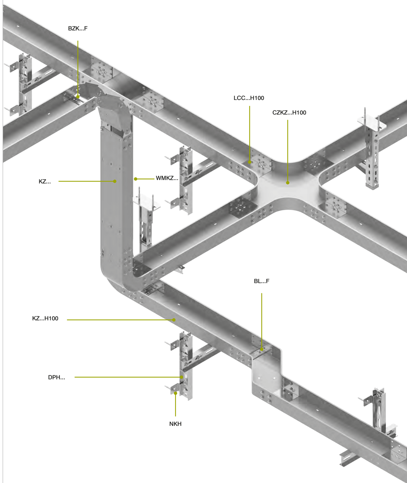
Ein Beispiel einer Kabeltrasseverlegung -Schwerlastsystem
